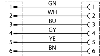
Devre şeması
