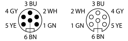
Devre şeması
