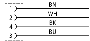
Devre şeması
