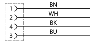
Devre şeması
