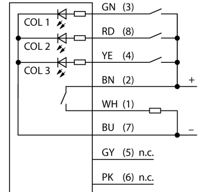
Kablo Bağlantı Şeması
