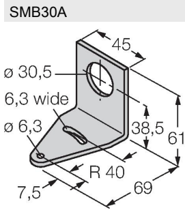
SMB30A 3032723 Montaj braket, dikdörtgen paslanmaz çelik, 30 mm dişli sensörler için
