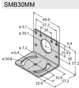
SMB30MM 3027162 Montaj braket, dikdörtgen paslanmaz çelik, 30 mm dişli sensörler için, hassas hizalama için geniş delikler
