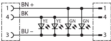
схема
