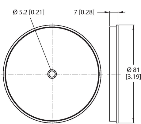
Чертеж с размерами Тип ID №
