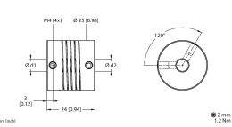
Cuplaj elicoidal din aluminiu Ø 25 mm; d1 = 6 mm, d2 = 10 mm
