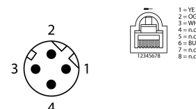
Schema de conexiuni
