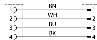
schemat obwodu
