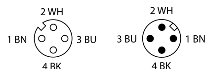
schemat obwodu
