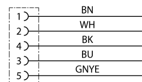
schemat obwodu
