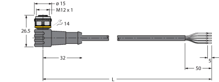
Rysunek wymiarowy Typ Nr kat.
