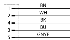
schakelplan
