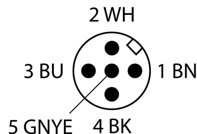
schakelplan
