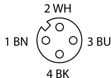
schakelplan
