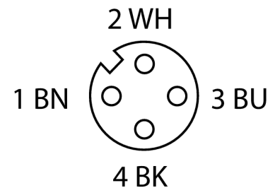
schakelplan
