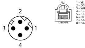
schakelplan
