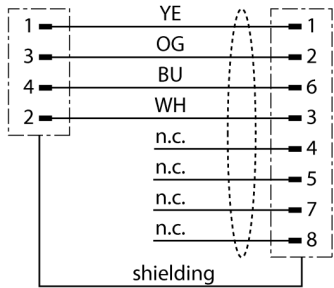
schakelplan
