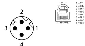
schakelplan
