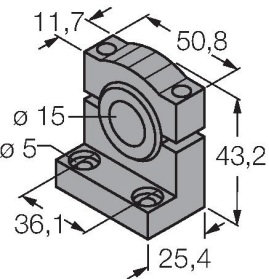
montagebeugel, PBT-zwart, voor PICO-GUARD Points
