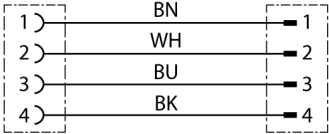
schéma de connexions
