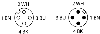
schéma de connexions
