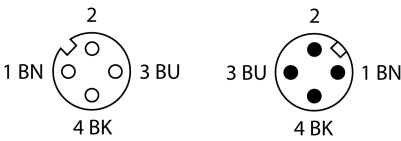
schéma de connexions
