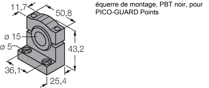
SMB18FM 3079421
