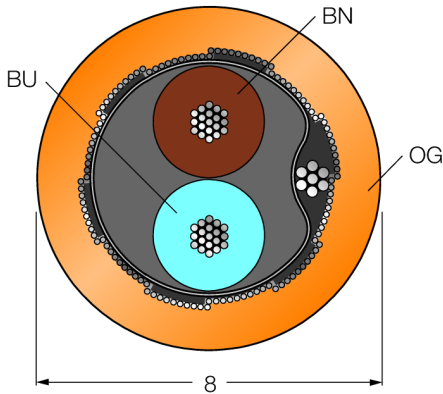
Sección transversal del cable
