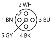
diagrama de conexiones
