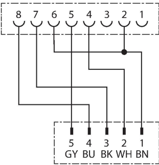
diagrama de conexiones
