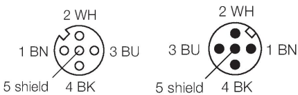
diagrama de conexiones
