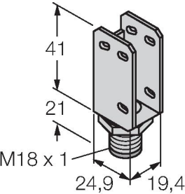
SMB18A 3033200 Soporte de montaje, en ángulo recto, acero inoxidable, para sensores con rosca de 18mm
