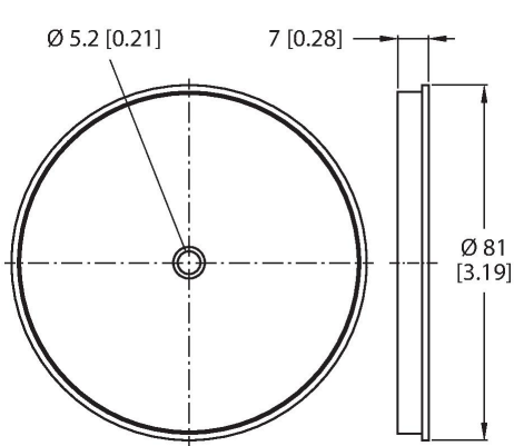
Dibujo acotado Tipo N.º de ID
