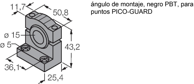
SMB18FM 3079421
