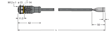
Dibujo acotado Tipo N.º de ID RKC4.4T-2/TEL 6625013
