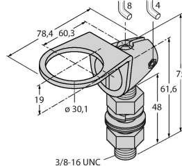
SMB30FA
