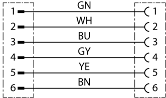
Schaltplan
