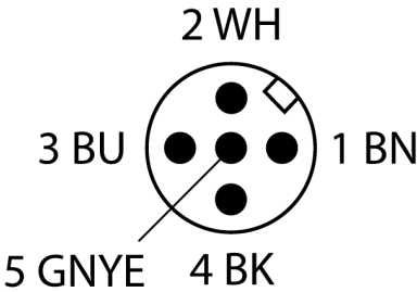
Schaltplan
