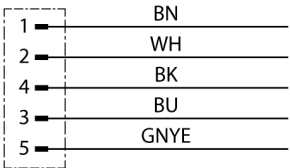
Schaltplan
