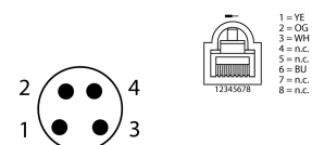
Schaltplan
