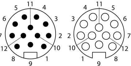
Schéma zapojení
