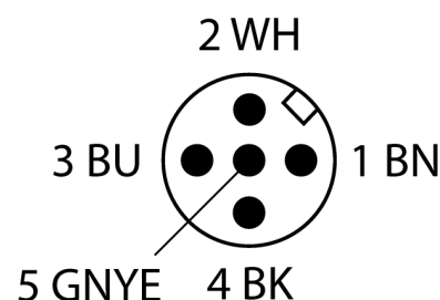
Schéma zapojení
