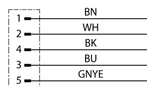
Schéma zapojení
