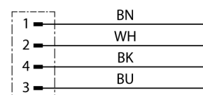
Schéma zapojení
