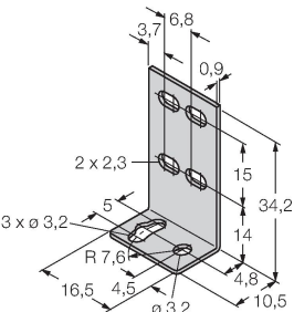
Montážní úchytka, materiál VA 1.4401, pro optosenzory Q12
