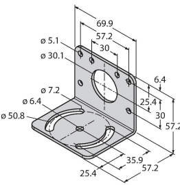
SMB30MM 3027162
