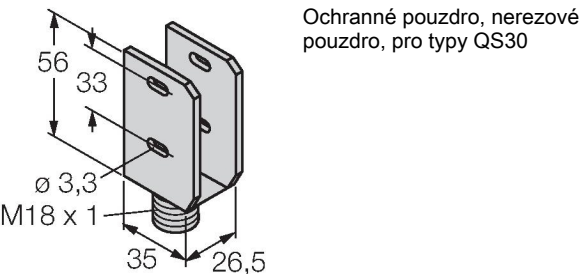
SMBQS30Y 3002811
