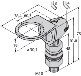
Montážní úchytka, nerez, pro závity 30 mm, závit M10 x 1,5
