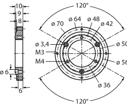
RFA-11 1544640 铝制法兰, 轴型夹紧法兰, Ø 70 mm; 厚10 mm, 适配Ø 70 mm法兰
