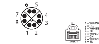
电路图
