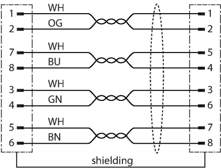
电路图
