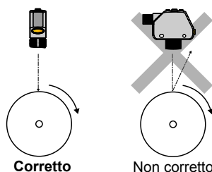
Figura 10. Orientamento per bersaglio altamente riflettente 1
