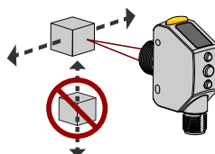
Figura 5. Orientamento ottimale del bersaglio rispetto al sensore
