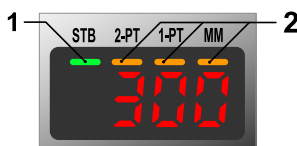
Figura 3. Display in modalità Run
