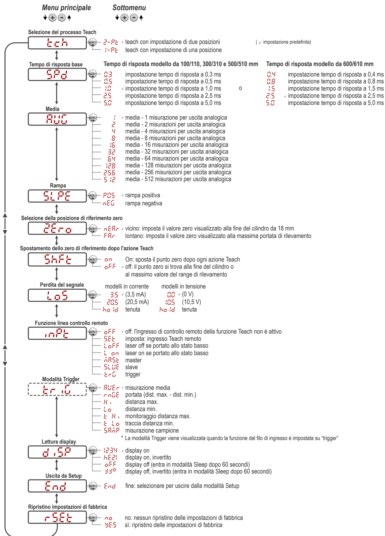
Figura 12. Menu sensore - Mappa
